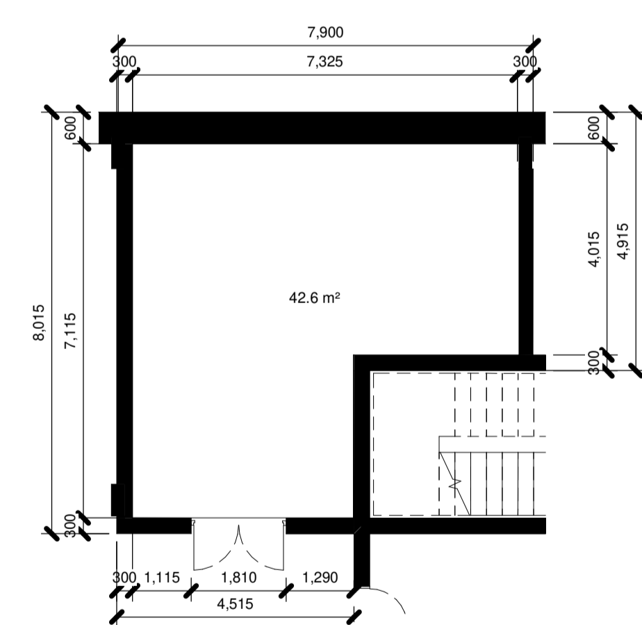
Refuse Block G Plan 1 : 100
