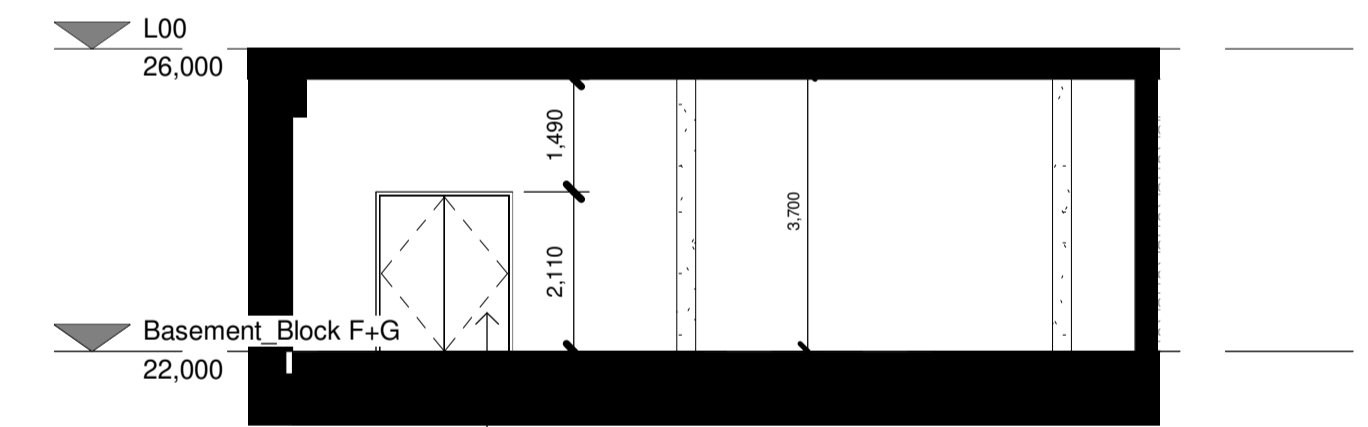
Refuse Block F Section 1 : 100
