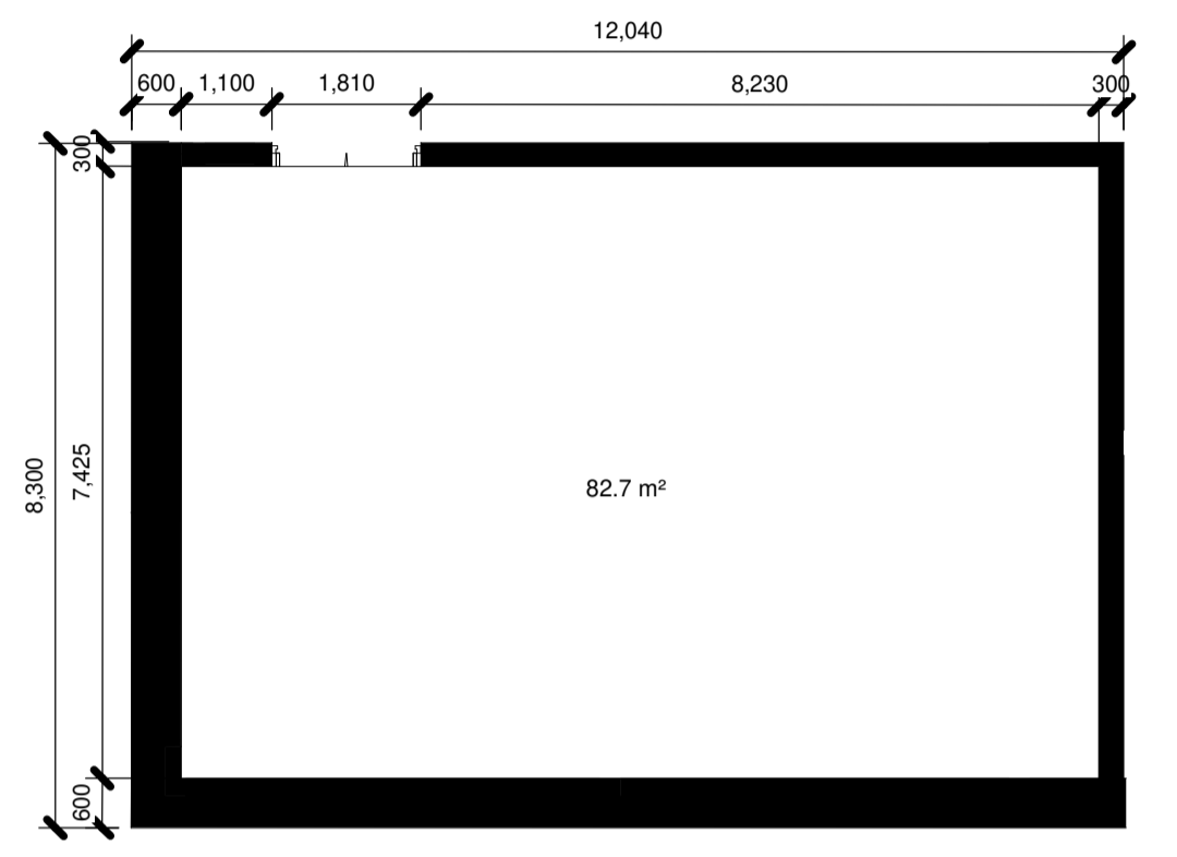
Refuse Block F Plan 1 : 100
